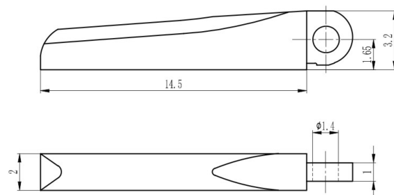
组合弹簧盒 Spring hinge XFP705EA20/W
