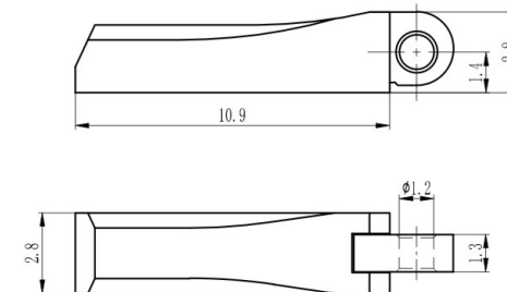
组合弹簧盒 Spring hinge XDF4009A28-Y
